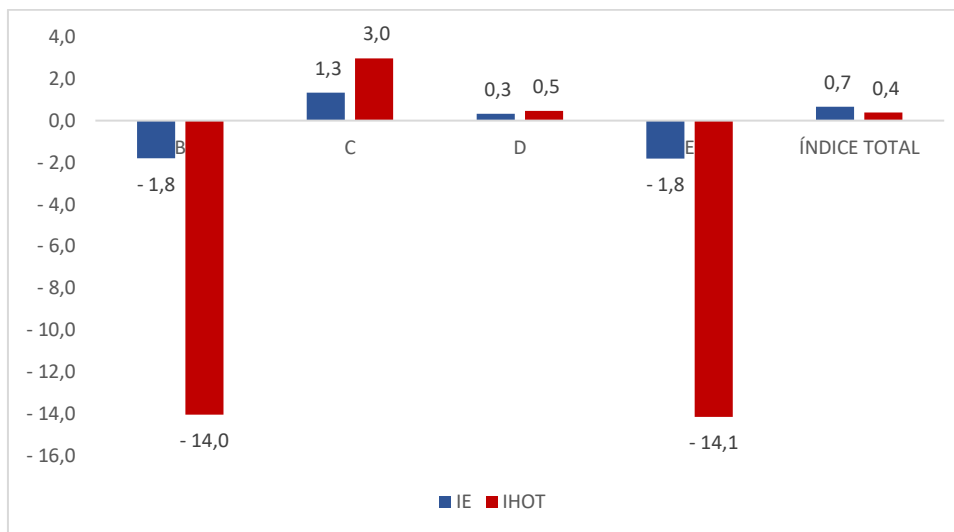
Gráfico 6 - Variações Homólogas do índice de Emprego e Horas Trabalhadas na indústria, total e por secção, %
